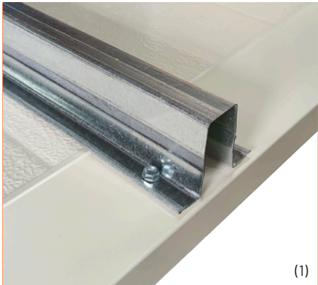
(1) Omega de refuerzo galvanizado
