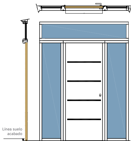
Detalle sistema de unión de puerta con lateral o dintel
